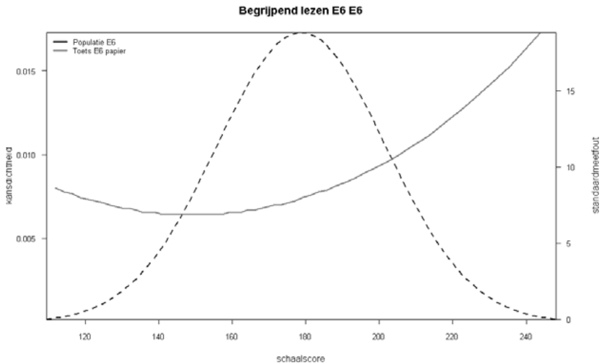
Figuur 5.2 Grootte van de meetfouten voor de toets E6 en de kansdichtheidsfunctie voor de E6-populatie
