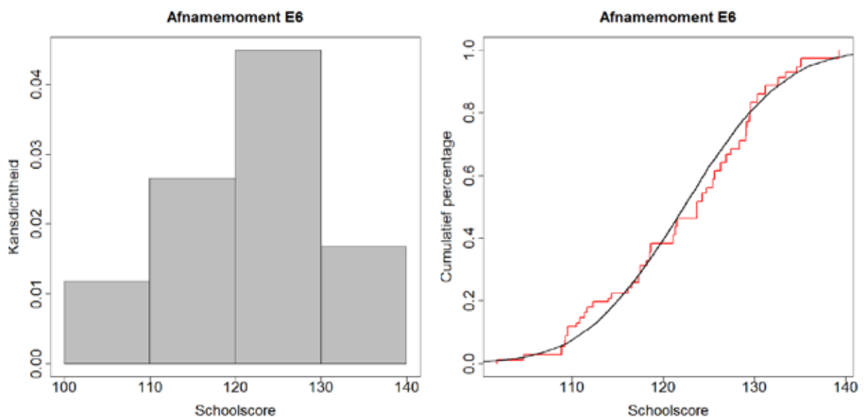
Figuur 4.8 Verdeling van de schoolgemiddelden voor LVS 3.0 Begrijpend lezen E6
