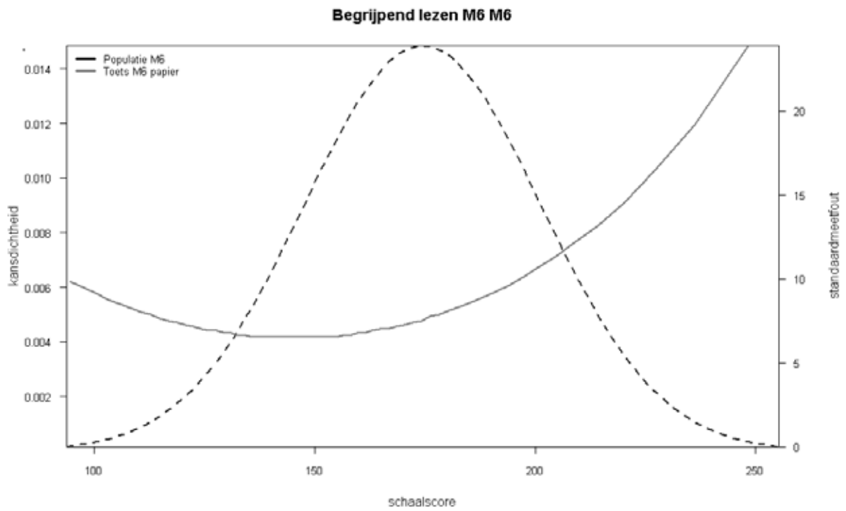
Figuur 5.1 Grootte van de meetfouten voor de toets M6 en de kansdichtheidsfunctie voor de M6-populatie
