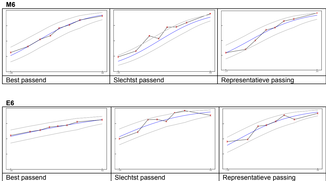
Figuur 4.6 Voorbeelden van S-toetsen voor de Toets LVS 3.0 Begrijpend lezen M6 en E6 met de best passende, de slechtst passende en een qua passing representatieve opgave
