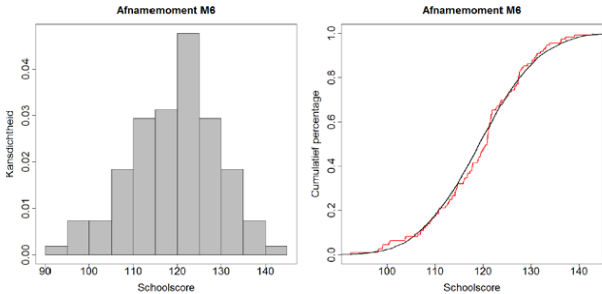
Figuur 4.7 Verdeling van de schoolgemiddelden voor LVS 3.0 Begrijpend lezen M6
